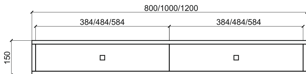
Вид спереди
